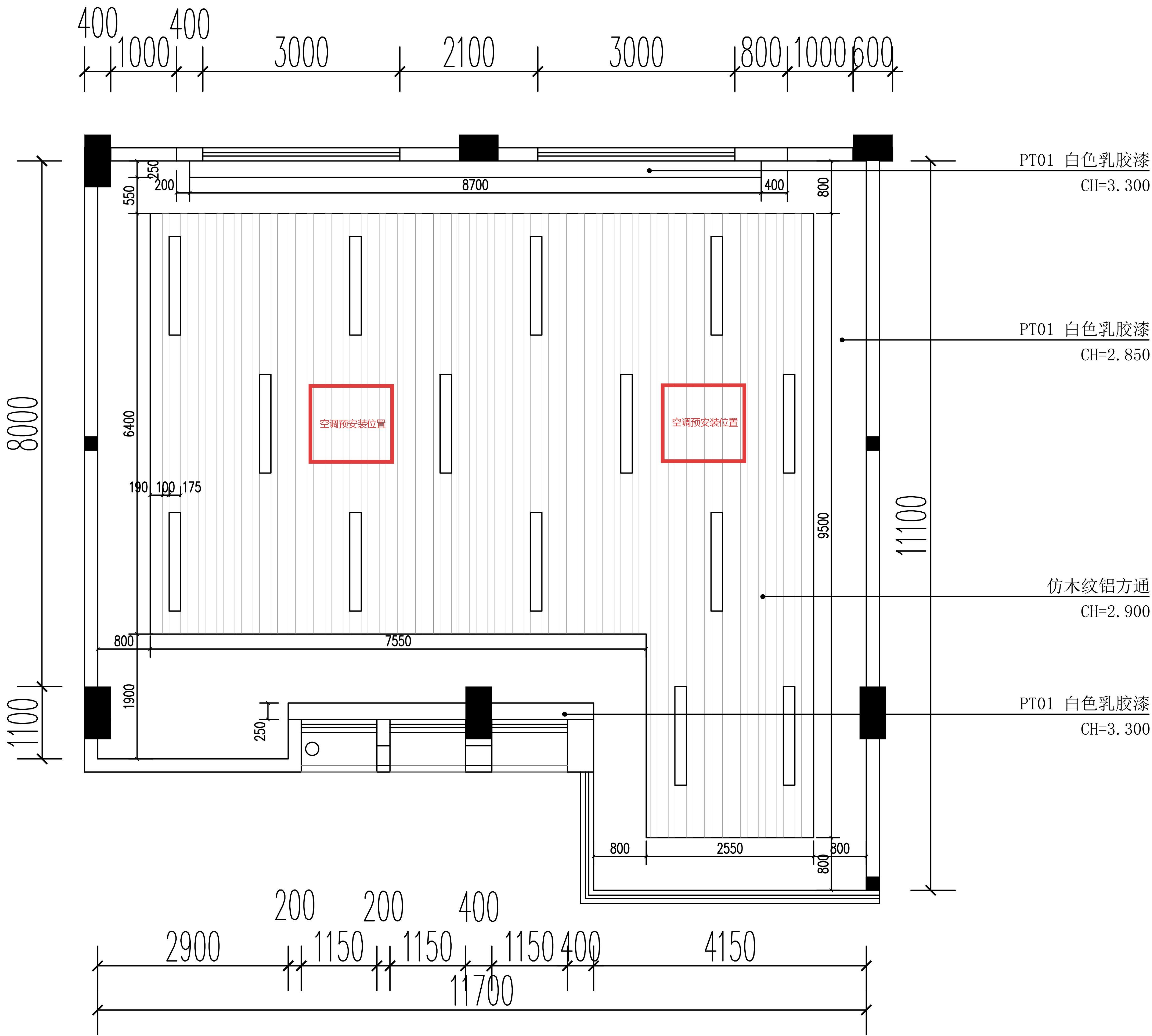
第一实训楼419天花布置图 1:70
