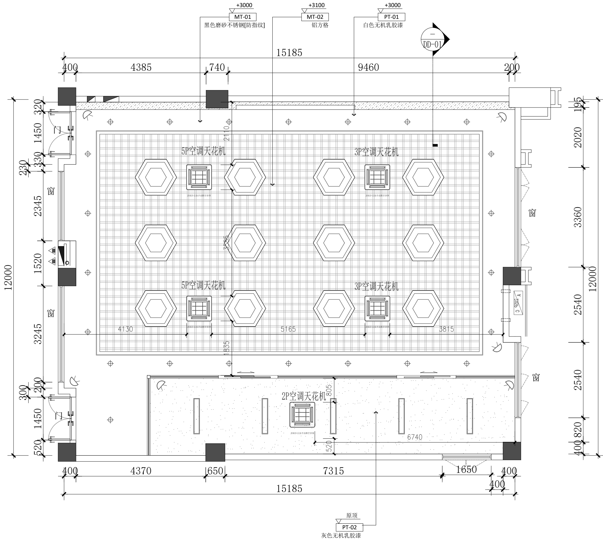
第二实训楼504天花综合图
